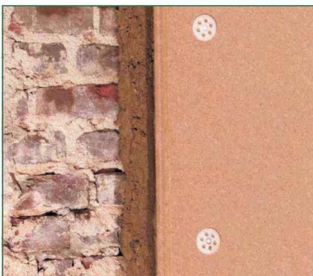
Na-isoleren aan de binnenzijde met leem en houtvezelisolatieplaat. Bron: Pavatex
