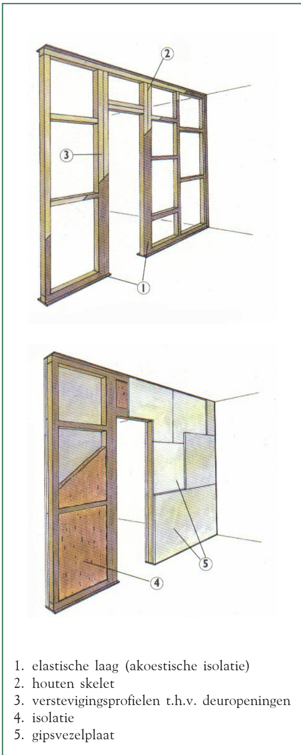
Constructie van een akoestisch geïsoleerde binnenwand. Bron: Lisolation phonique ecologique, terre vivante
