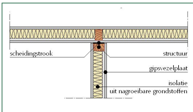
Figuur 4.5: Aansluiting muur-muur, T-verbinding
