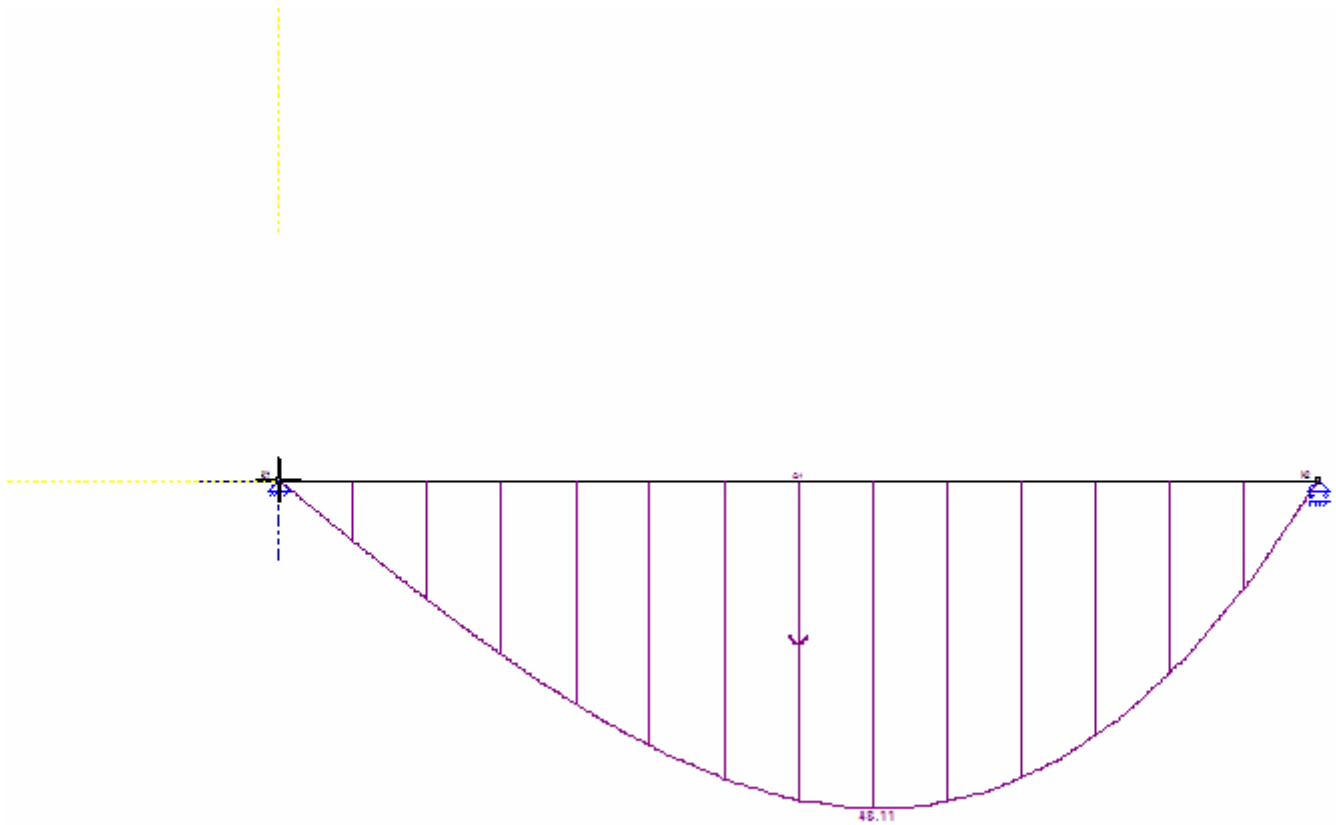
Afb. N-lijn BG1
