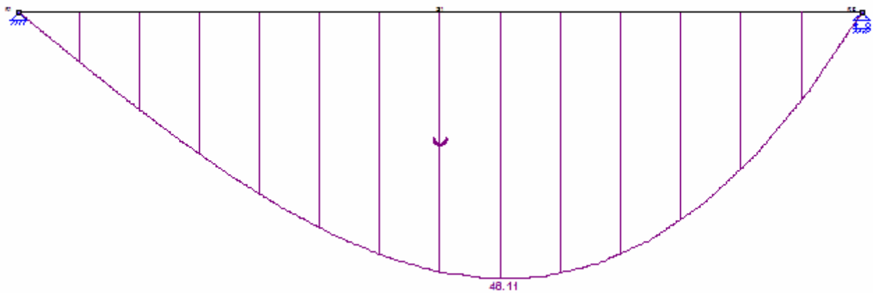
Afb. M-lijn BG1
