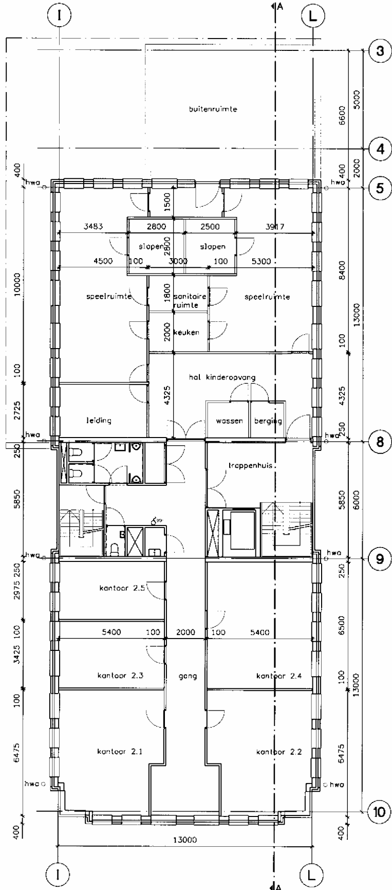
figuur 6.24 - Tweede verdieping van bouwplan 3 (schaal 1:200)
