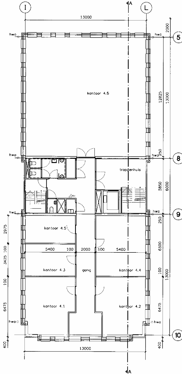
figuur 6.26 - Vierde verdieping van bouwplan 3 (schaal 1:200)
